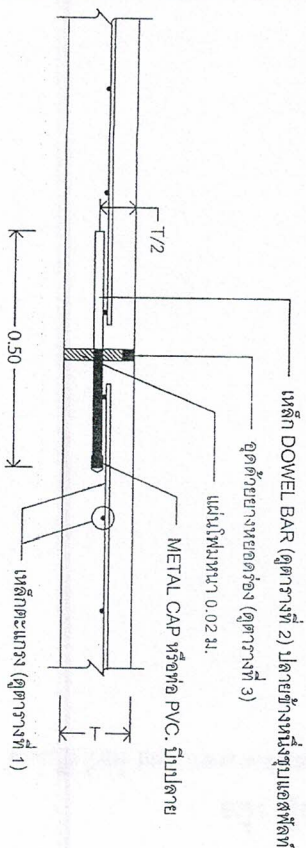
EXPANSION JOINT (ขนาด 100 มม.)
