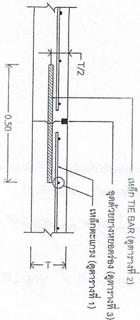
LONGITUDINAL JOINT (ຕາມການເກາະຂອງຄ່າມ ຄູ່ຂຶ້ນ)
